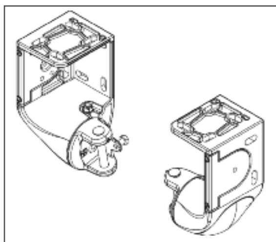
coppia supporti
