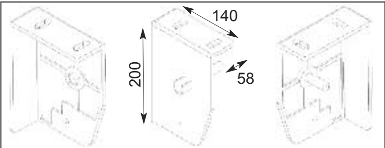
supporti in alluminio estruso
