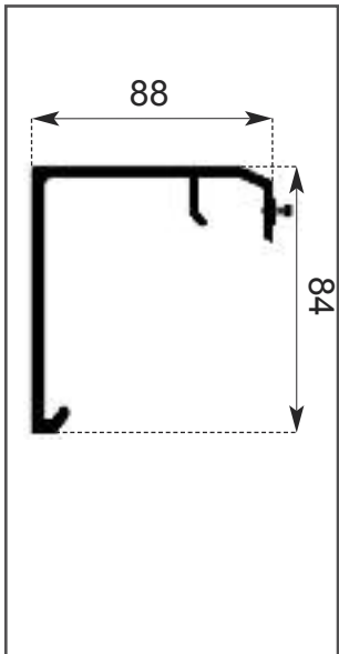
PIASTRA ATTACCO PARETE
