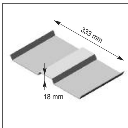
COPRIGUIDA VERNICIATO TMA Disponibile 4/5/6 mt € 31,00 ml
