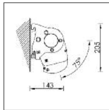
montaggio a parete 75°
