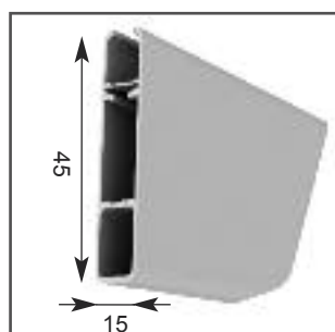
profilo 45
