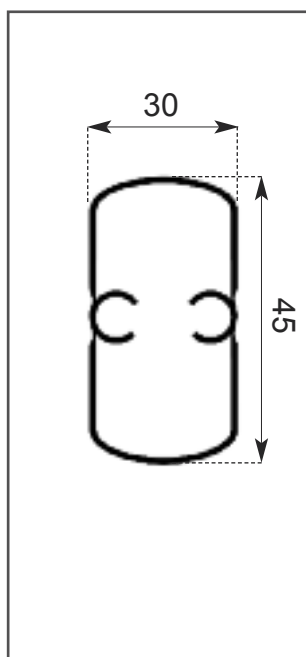
BRACCETTO
