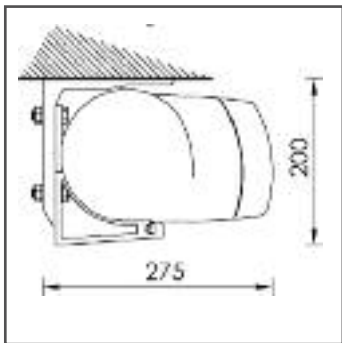
montaggio a soffitto
