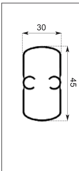
BRACCETTO
