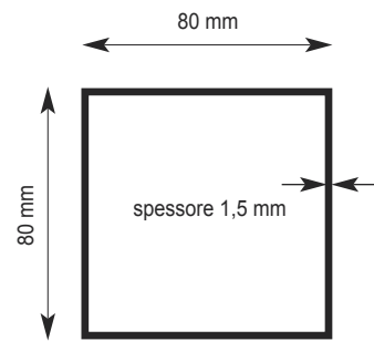
Sezione Montante
