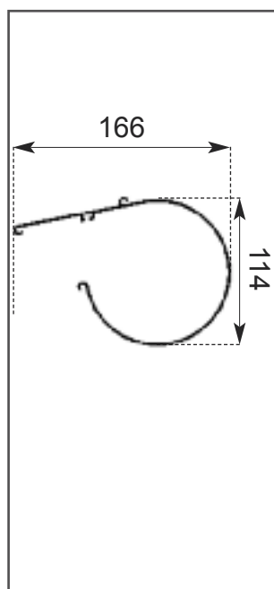
CASSONETTO IN ALLUMINIO ESTRUSO
