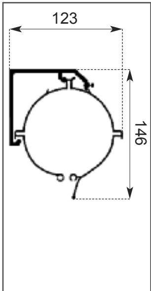
PIASTRA + CASSONETTO (attacco a parete)
