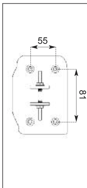
PIEDINO IN ALLUMINIO
