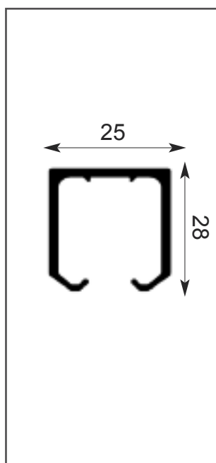
PROFILO GUIDA
