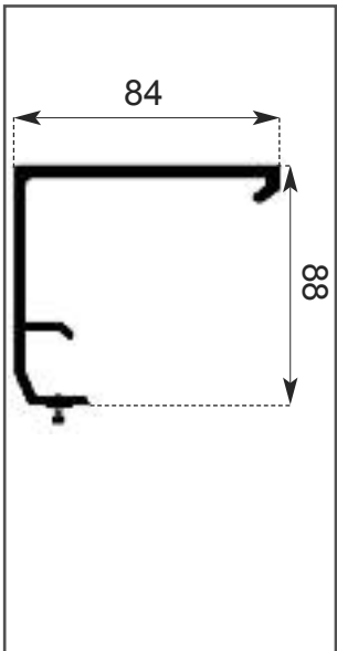
PIASTRA ATTACCO SOFFITTO
