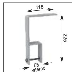
supporto tettino ( 22,80 cad.)
