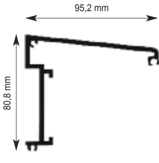
Gronda a muro (Obbligatoria)
