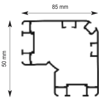
Gamba angolare
