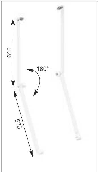
braccetti rotanti (180°)
