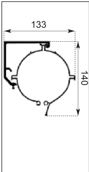
PIASTRA + CASSONETTO (attacco a soffitto)
