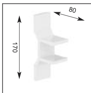
staffa a parete in alluminio estruso (di serie)
