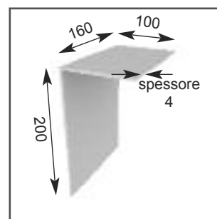
piastra attacco spallina spigoli al vivo (fornita senza fori) -
