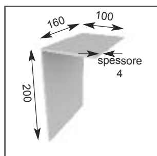
piastra attacco spallina spigoli al vivo (fornita senza fori) - € 40,50 cp.
