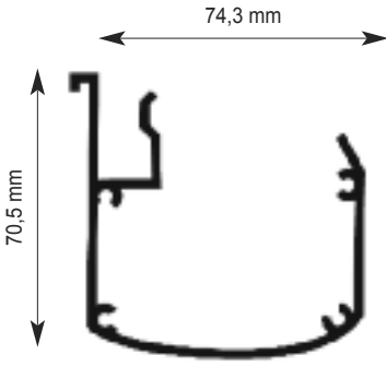
Gronda laterale
