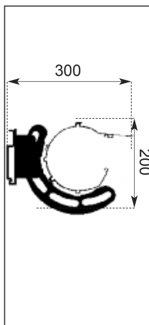
CASSONETTO IN ALLUMINIO ESTRUSO CON STAFFA
