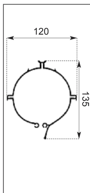
CASSONETTO
