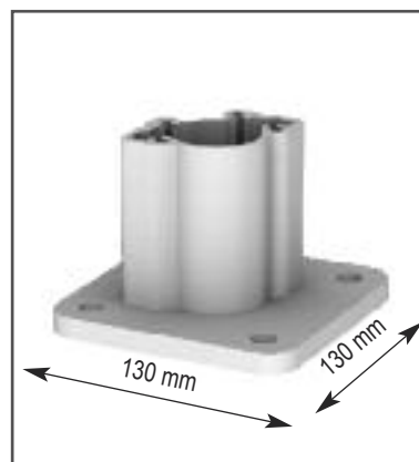
Piede per gamba ad angolo
