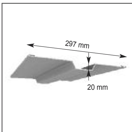
COPRIGUIDA VERNICIATO TMG Disponibile 4/5/6 mt € 31,80 ml
