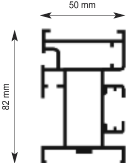
Trave portante
