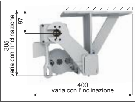
ingombri attacco a soffitto
