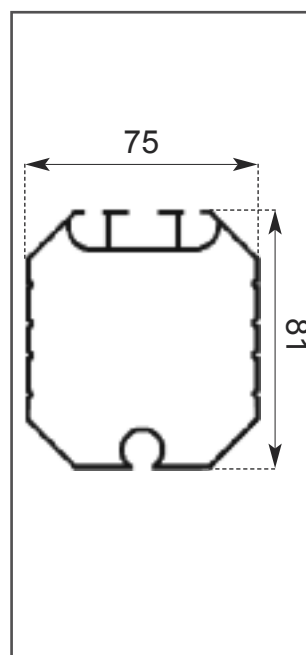
TERMINALE IN ALLUMINIO ESTRUSO
