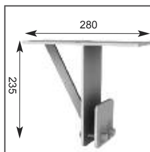
staffa opzionale con supplemento (attacco a soffitto)
