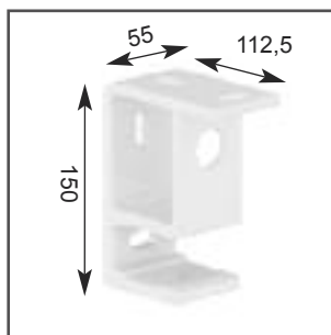
supporto in alluminio estruso parete/soffitto
