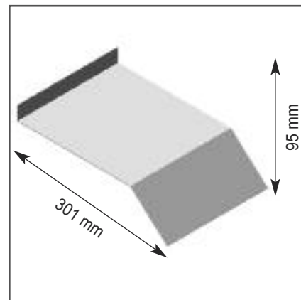
TETTINO CON ALETTA VERNICIATO TBQ E TMA Disponibile 4/5/6 mt € 31,00 ml
