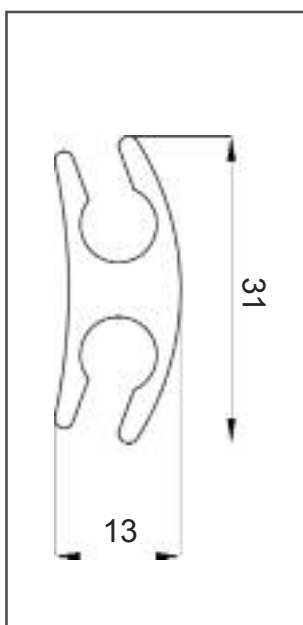
PROFILO DI RINFORZO
