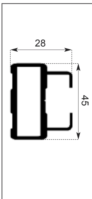
GUIDA IN ALLUMINIO TMG ESTRUSO
