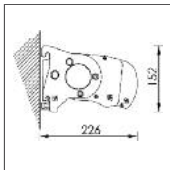
montaggio a parete 0°
