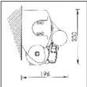
INSTALLAZIONE A PARETE
