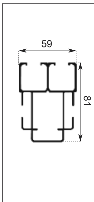
GUIDA IN ALLUMINIO ESTRUSO
