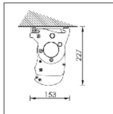
montaggio a soffitto 90°
