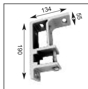
supporto in alluminio estruso parete/soffitto (a richiesta)
