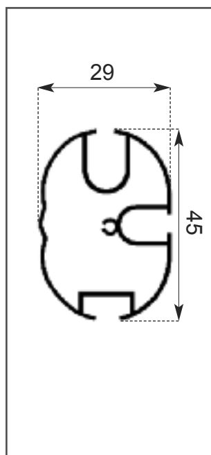
PROFILO FRANGITRATTA
