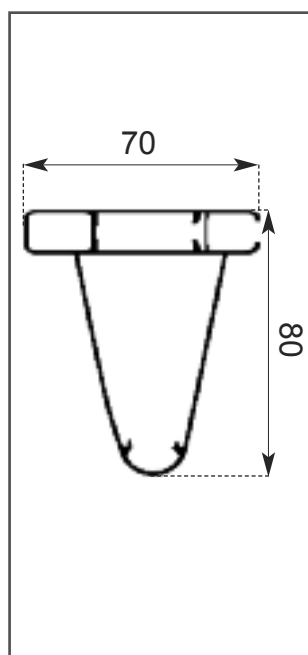
PROFILO TERMINALE DA 70 RINFORZATO
