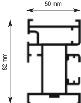
Trave portante
