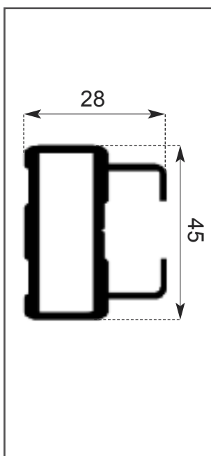
GUIDA IN ALLUMINIO ESTRUSO
