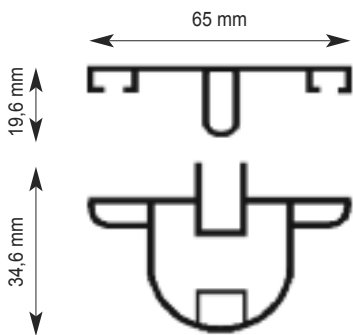
Supporto
