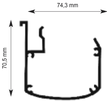
Gronda laterale
