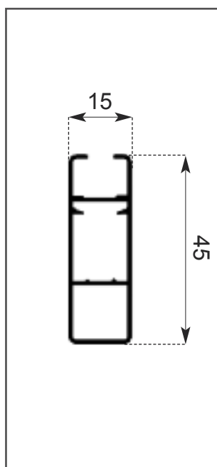
PROFILO 45
