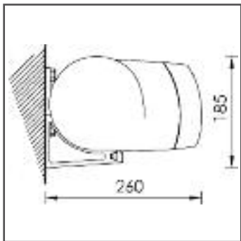
montaggio a parete
