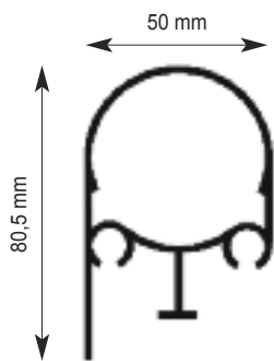
Trave perimetrale
