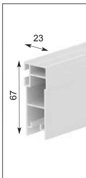
GUIDA
