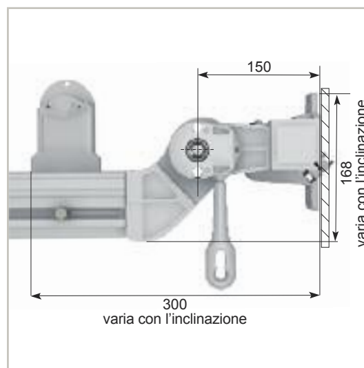
INGOMBRI ATTACCO A PARETE
