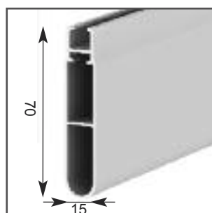
profilo centina da 70 intermedio
