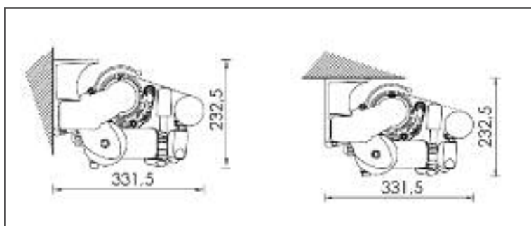
TERMINALE IN ALLUMINIO ESTRUSO
