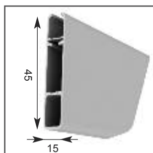
profilo 45
