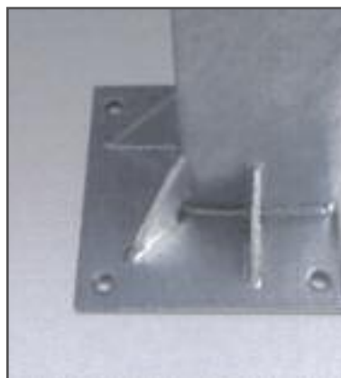
Piastra base
