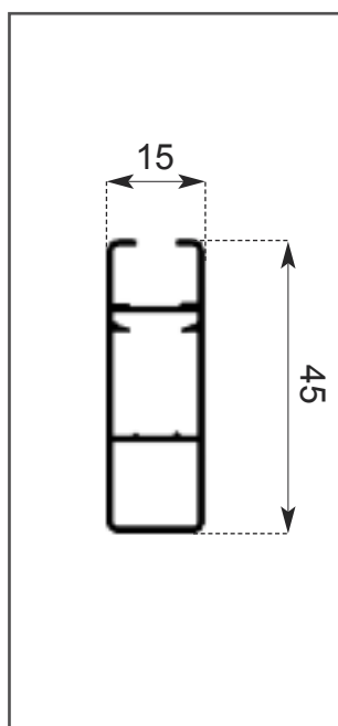
PROFILO 45
