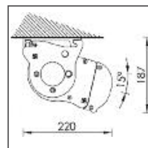
montaggio a soffitto 15°
