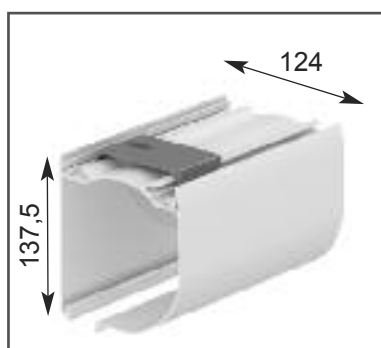
CASSONETTO
