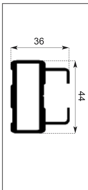
GUIDA TMG
